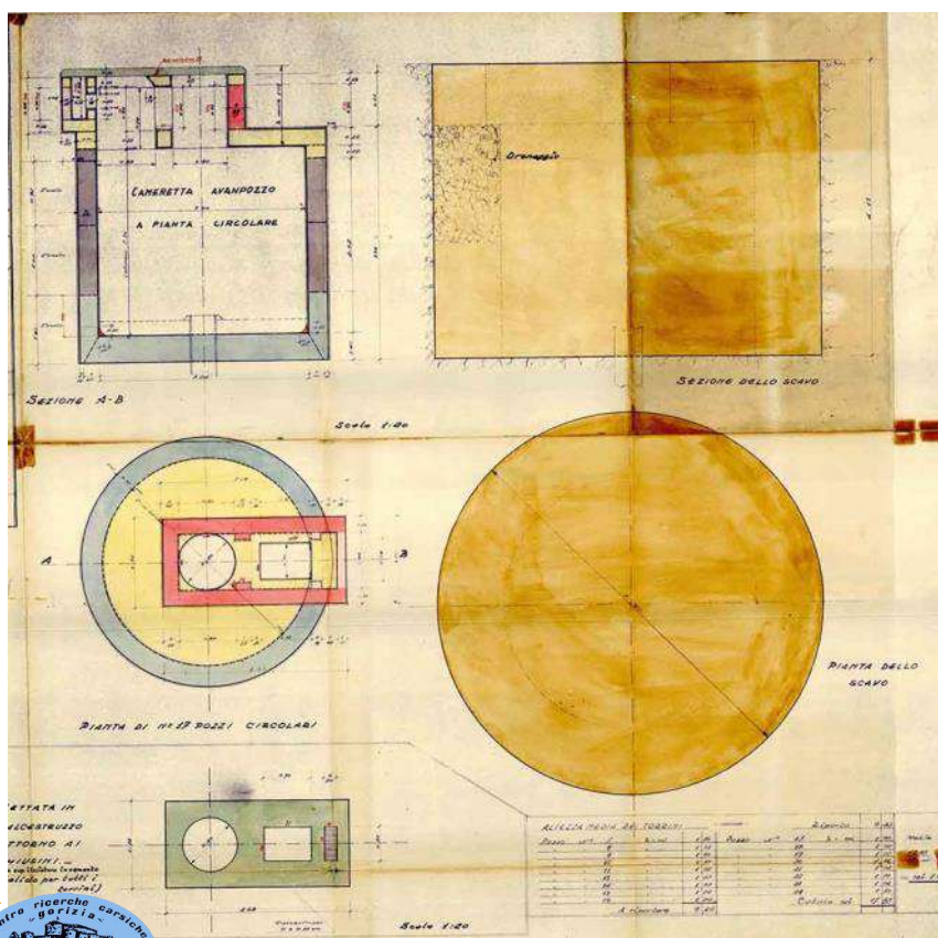
Fig. 88. Centrale di pompaggio San Siro: «Cameretta dell'avampozzo n° 12» (Cittadella degli Archivi e Archivio Civico Milano).
