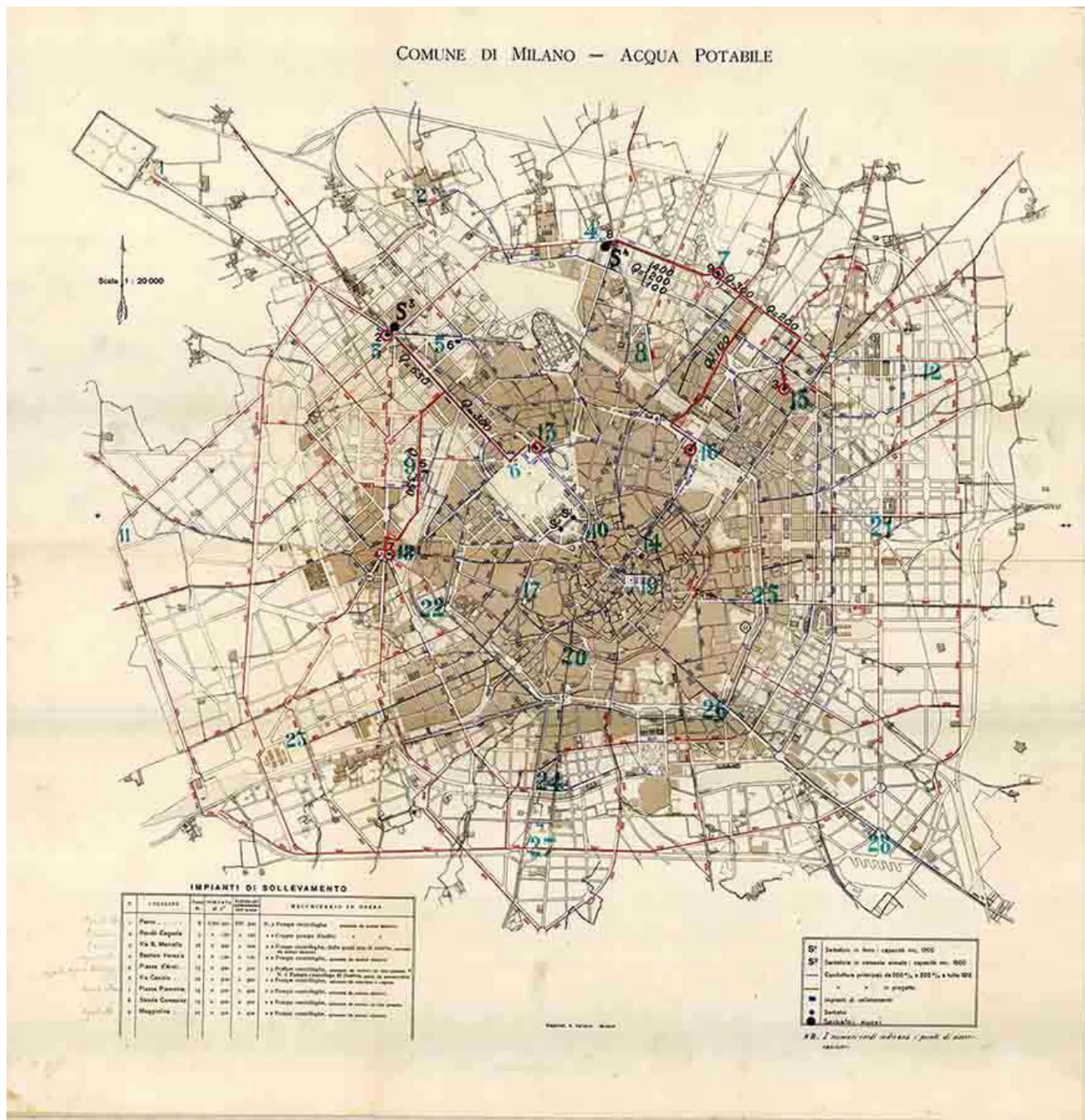
Fig. 38. Planimetria della rete d'acquedotto al 1912. Con tratto blu è indicata la rete principale esistente (tubazioni di diametro compreso tra i 200 e i 600 mm), con tratto rosso è rappresentata la rete in progetto. Sono anche riportate le nove Centrali di pompaggio funzionanti e i due serbatoi realizzati nei Torrioni del Castello di Porta Giovia (Cittadella degli Archivi e Archivio Civico Milano).
