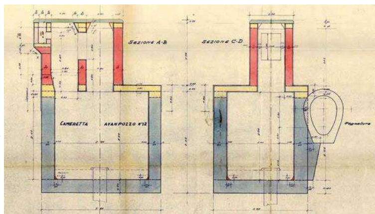
Fig. 88. Centrale di pompaggio San Siro: «Cameretta dell'avampozzo n° 12» (Cittadella degli Archivi e Archivio Civico Milano).
