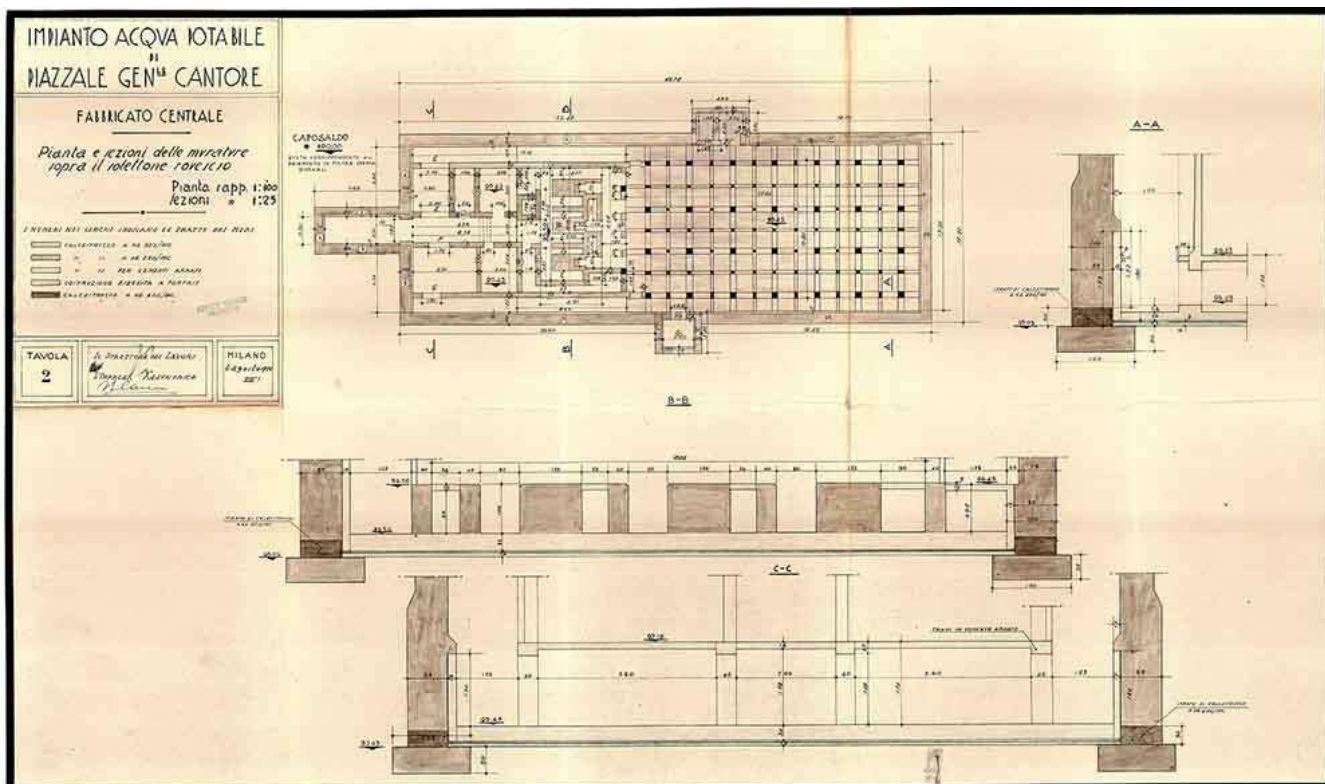
Fig. 81. Centrale di pompaggio Cantore: «Impianto acqua potabile di Piazzale Genle Cantore. Fabbricato centrale. Pianta e sezioni delle murature sopra il solettone rovescio»; disegno del 6 agosto 1935 (Cittadella degli Archivi e Archivio Civico Milano).
