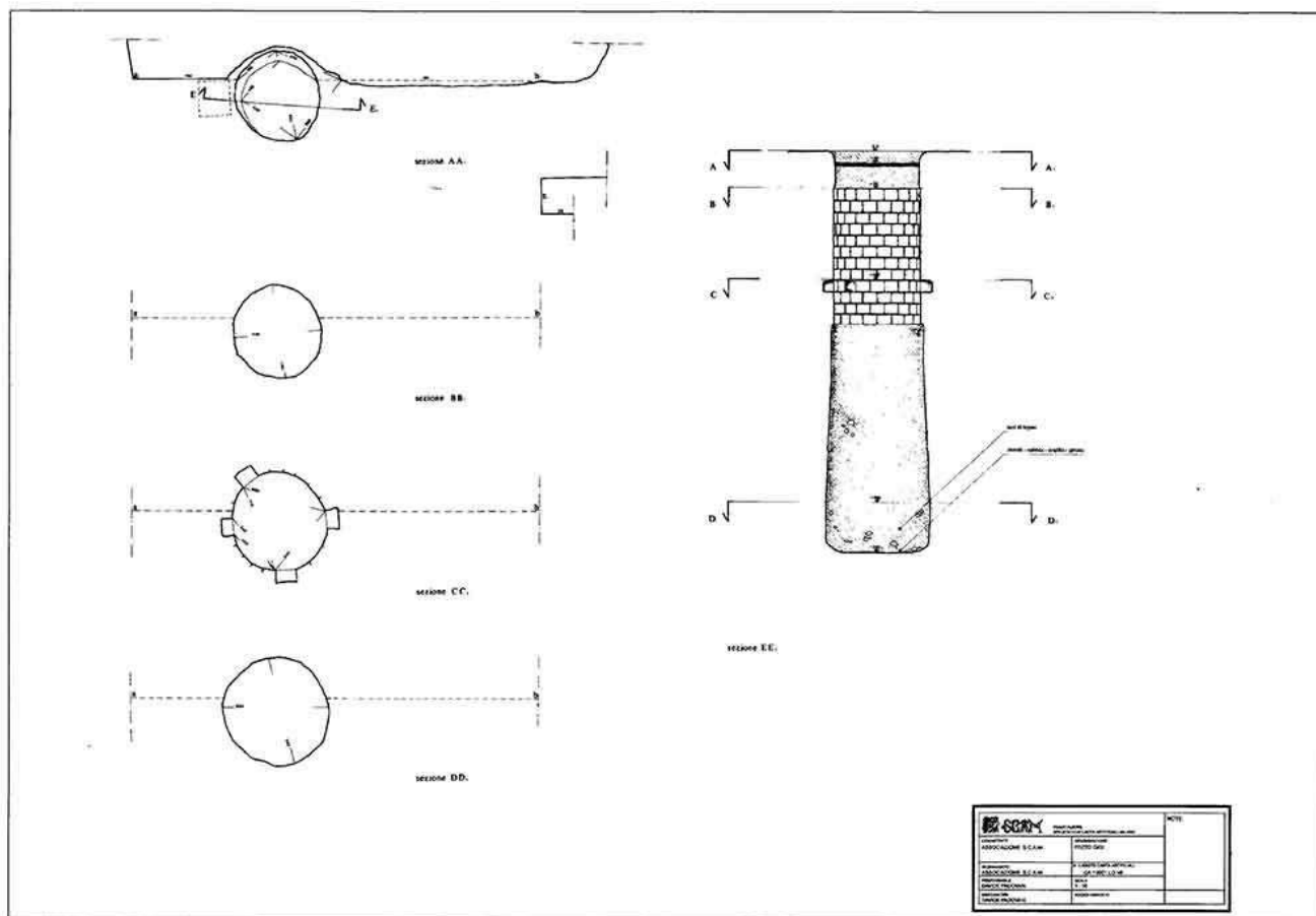
Fig. 17. Pozzo rilevato nei sotterranei della Chiesa di San Simpliciano a Milano dagli speleologi dell'Ass.ne S.C.A.M. (N° Catastale CA 10021 LO MI).
