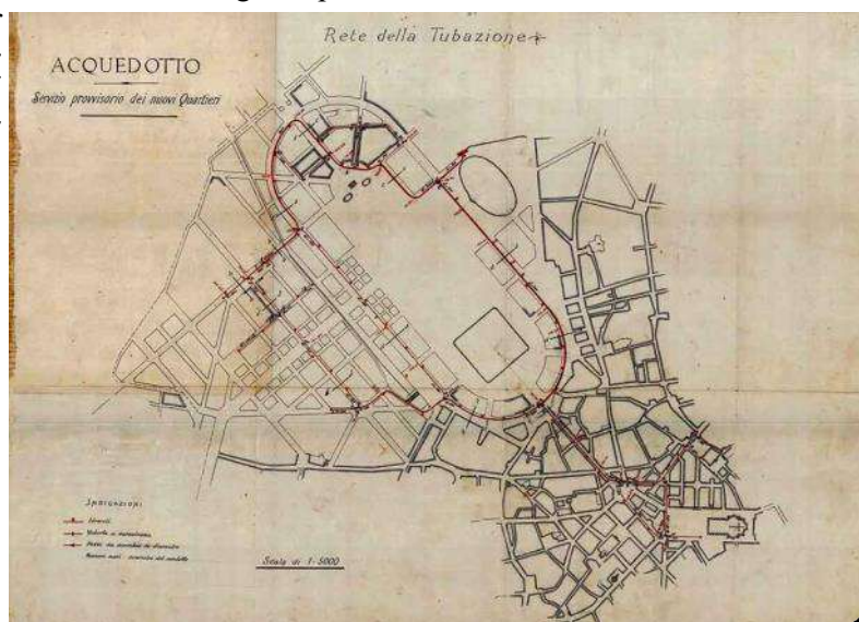
Fig. 29. Planimetria del 1888: «Rete delle Tubazione - Acquedotto - Servizio provvisorio dei nuovi Quartieri» (Cittadella degli Archivi e Archivio Civico Milano).
