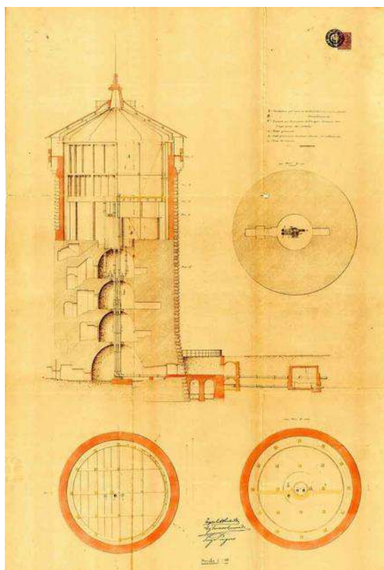
Fig. 34. Serbatoi in cemento realizzati all'interno del Torrione Sud del Castello di Porta Giovia. Tavola di inizio Novecento (Cittadella degli Archivi e Archivio Civico Milano).
