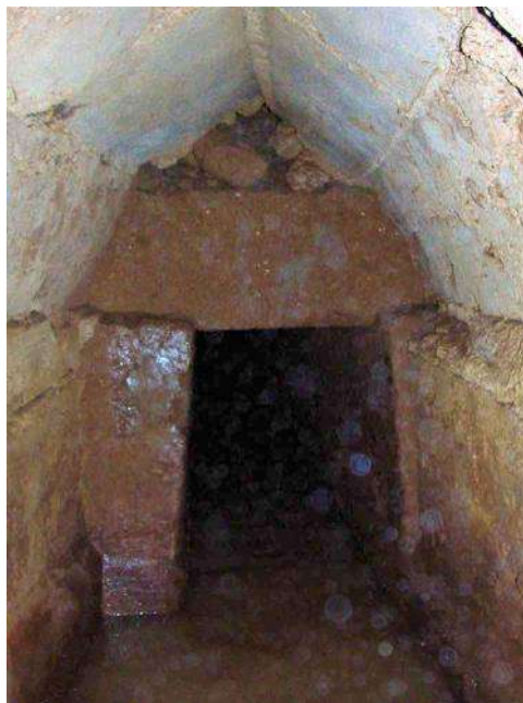
Fig. 15. Antico acquedotto ipogeo esplorato e rilevato nell'Agro Volsiniese (N° Catastale CA 00117 LA VT).
