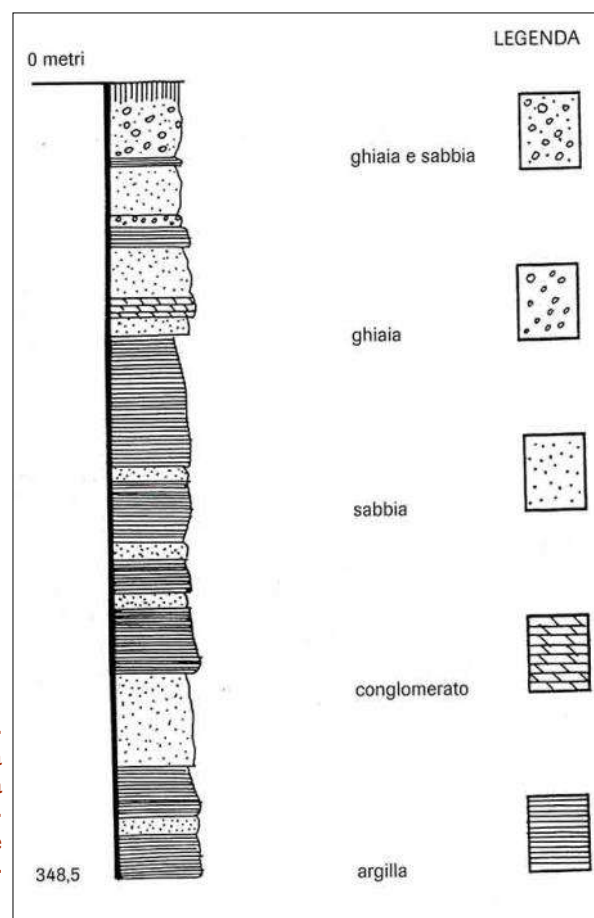
Fig. 8b. Sezione idrogeologica, rappresenta la struttura geologica superficiale del sottosuolo nell'area del Castello di Porta Giovia e la stratigrafia del pozzo dell'Arena Civica situato a nord est del Castello. La tavola è tratta da: Paolo Bassi, Roberto Berto, Fabrizio Perletti, Inquadramento geologico regionale del territorio di Milano, in Gianluca Padovan (a cura di), La forza celata, Diakronia, Vigevano 1996, pp. 28-30.
