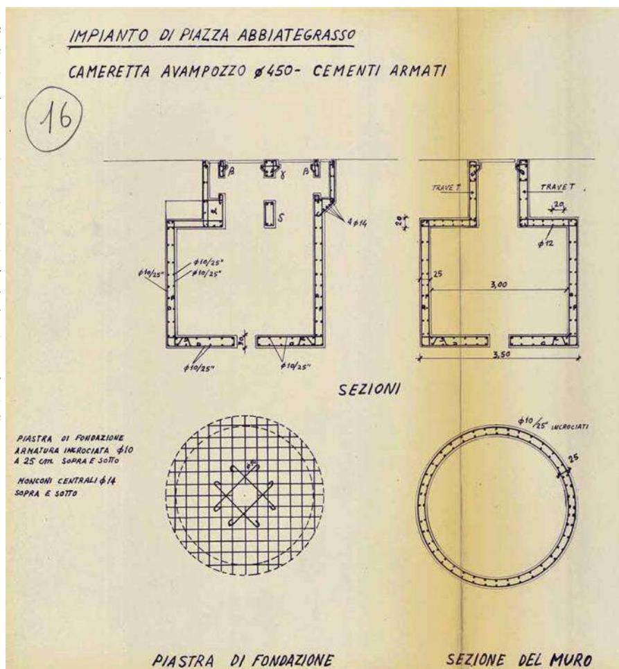
Fig. 97. Cameretta dell'avampozzo della Centrale di pompaggio Abbiategrasso (Cittadella degli Archivi e Archivio Civico Milano).
