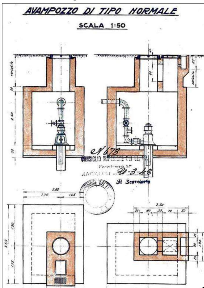
Fig. 79. 1948: avampo di tipo normale della Centrale di pompaggio Tonezza, chiamata anche Carriera in taluni documenti (Cittadella degli Archivi e Archivio Civico Milano).
